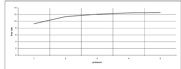
Diagrama de caudal - Flow rate curves - Diagramme de débit
